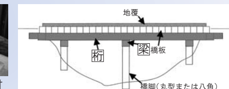
橋の梁材と桁材
